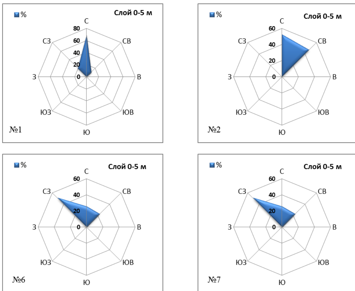
Рис. 3 Повторяемость течений по направлениям (%) в слое 0-5 м на восточной границе лицензионного участка «Северо-Каспийская площадь» 10 октября 2013 года
