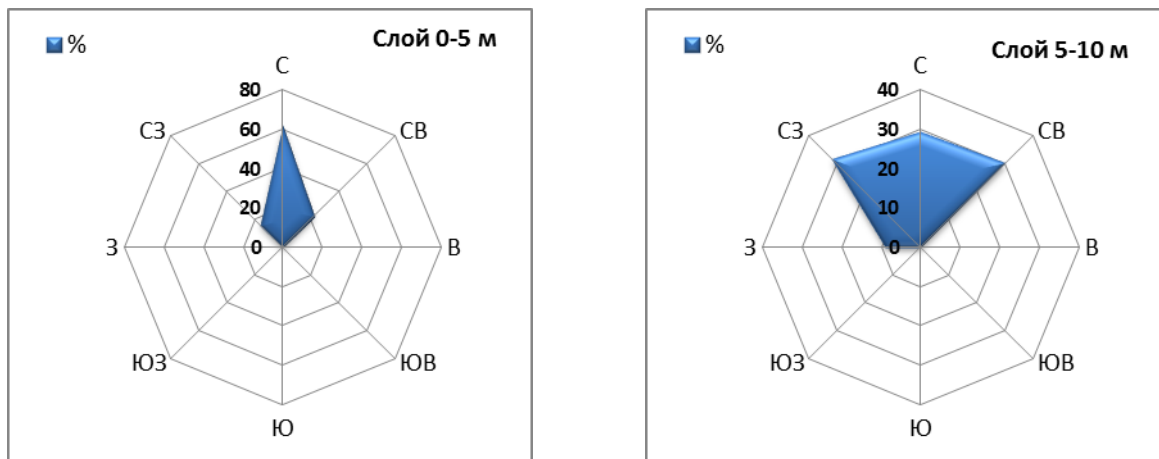
Рис. 2 Повторяемость течений по направлениям (%) на восточной границе лицензионного участка «Северо-Каспийская площадь» 10 октября 2013 года
