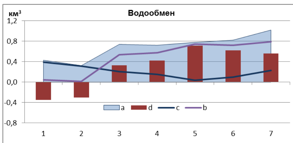
Рис. 4 Водообмен в различных секторах на восточной границе лицензионного участка «Северо-Каспийская площадь» 10 октября 2013 года в слое 0-10 метров. На оси абсцисс – номера секторов с севера на юг; a – суммарный водообмен; b – приток; c – отток; d – результирующий водообмен
