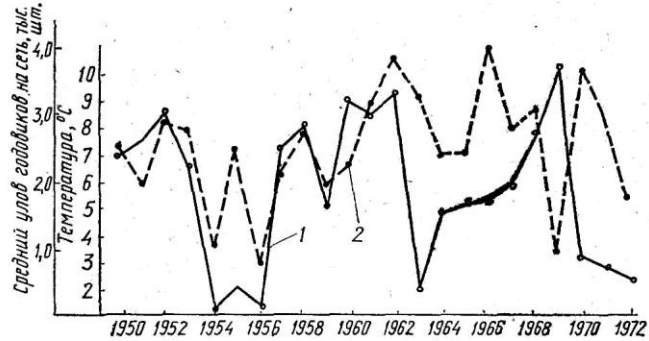
Рис. 2. Численность поколений анчоусовидной кильки (1) и средняя температура воздуха за январь — апрель по годам (2).
