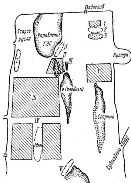
Схема расположения нерестилищ белорыбца в приплотинной зоне Волгоградской ГЭС:
